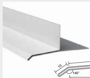
Horizontāla klājuma profils
